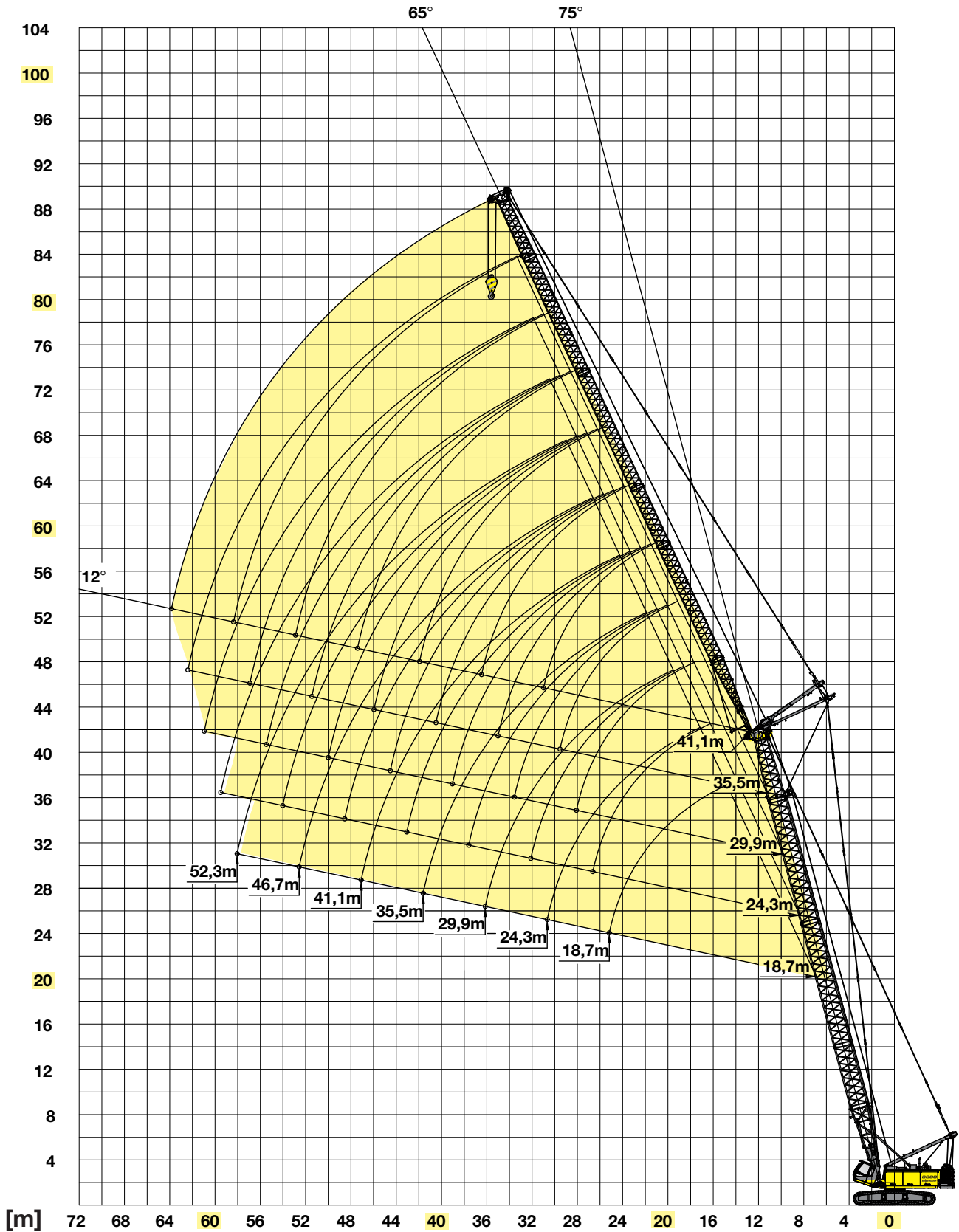
Auslegerzusammenbau siehe Seite 23 Boom configuration see page 23
